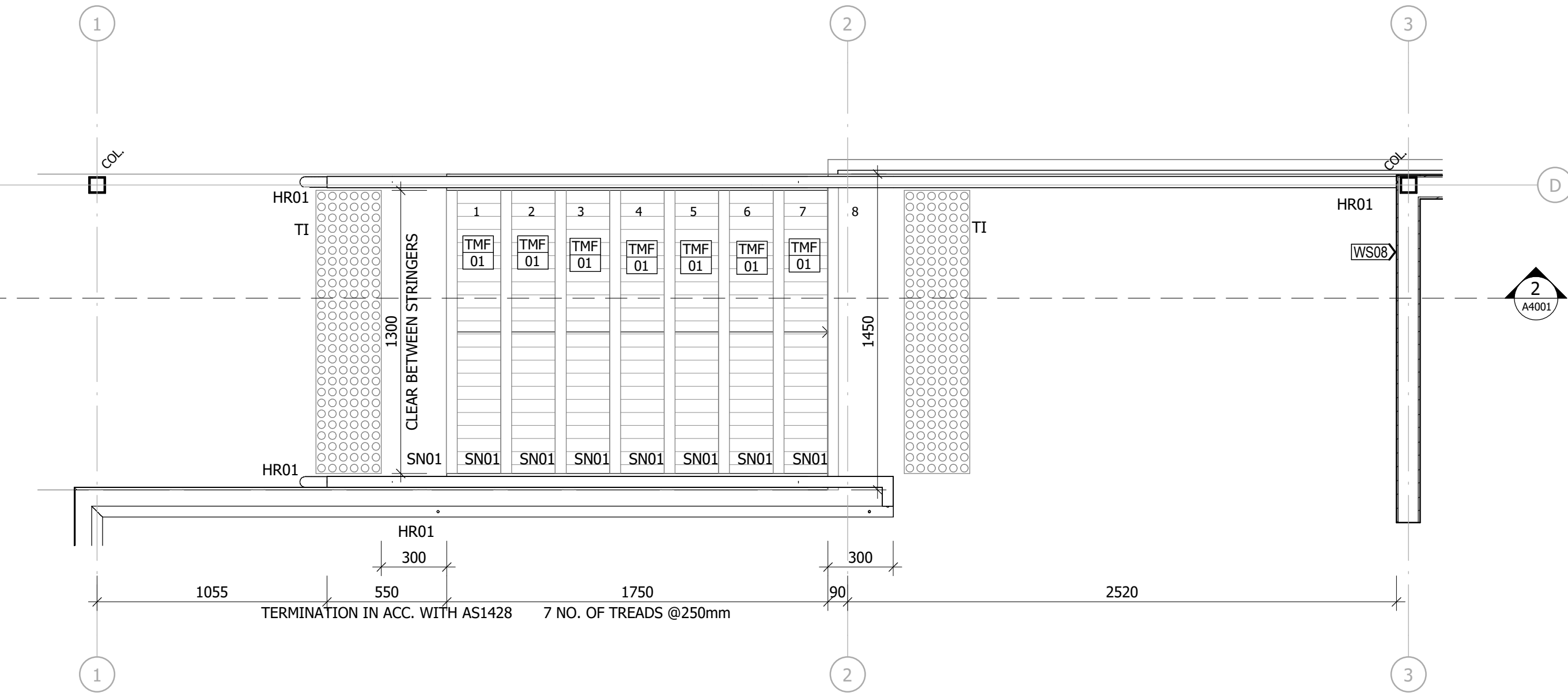
1 STAIR 1 - PLAN A2001/ 1 : 20
