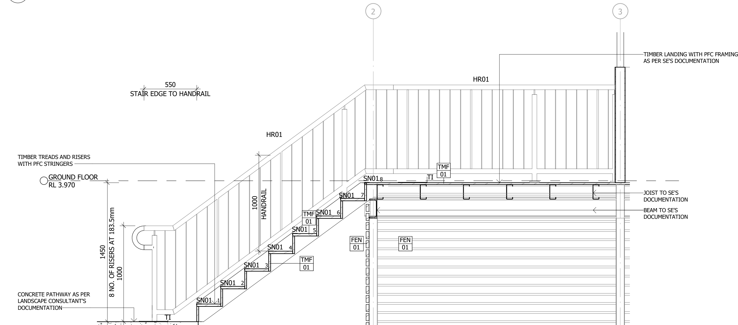
2 STAIR 1 - SECTION A4001/ 1 : 20
