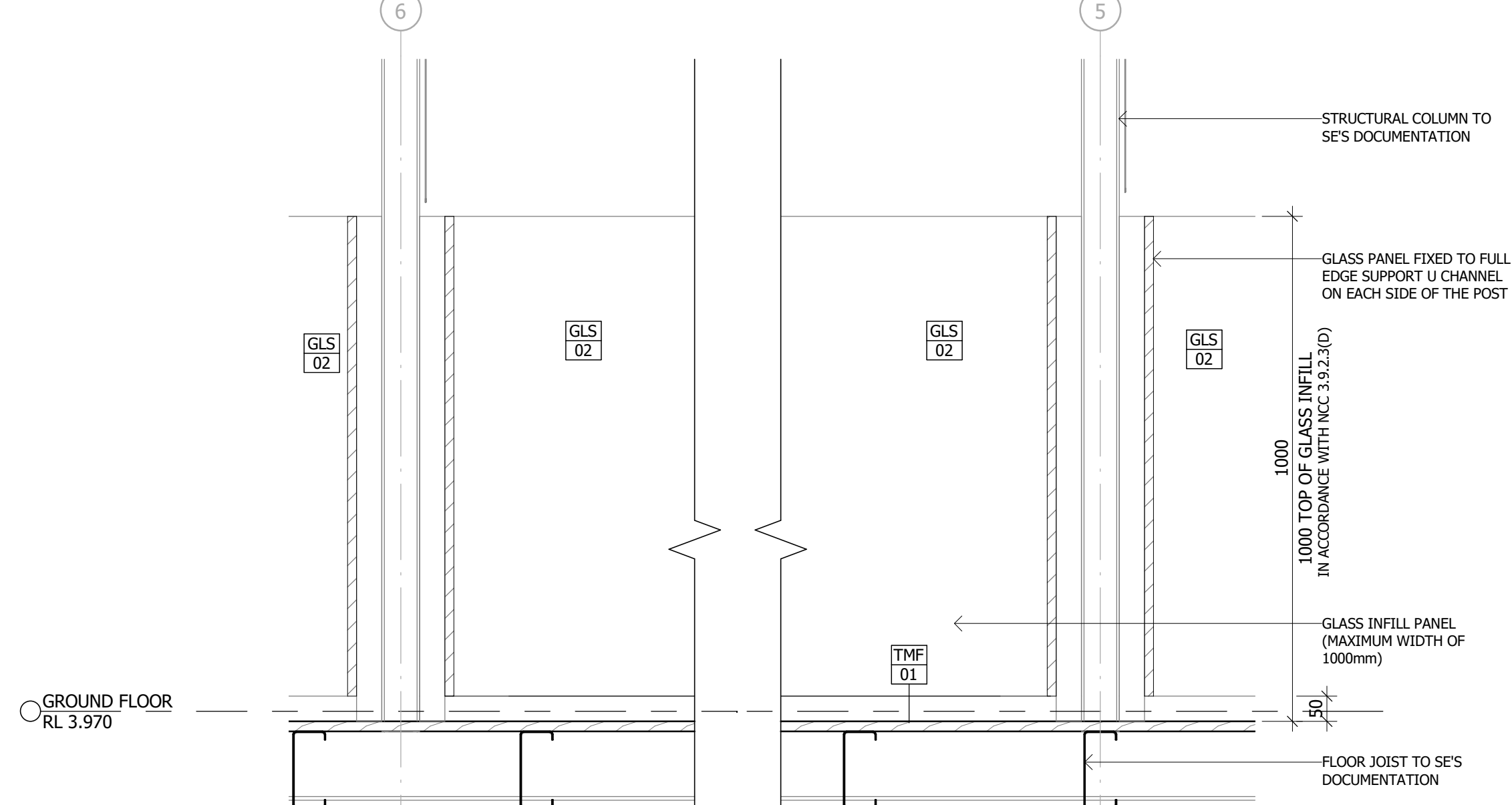
4 STAIR 2 - SECTION A4001/ 1 : 20
